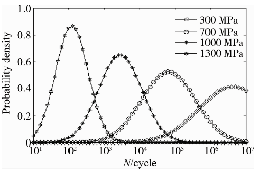
图 12 200\text{ }^\circ\text{C} 时不同应力下的寿命分布 Fig. 12 Life distribution with different stress at 200\text{ }^\circ\text{C}
