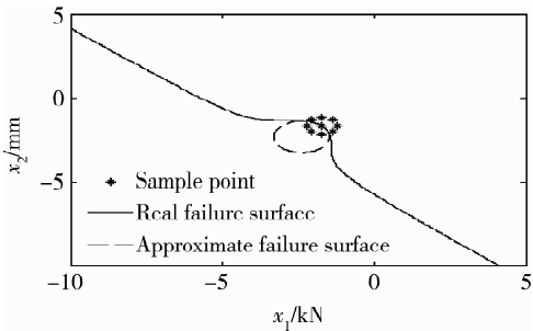
图 6 例 1 第 4 次迭代 Fig. 6 Fourth iterative step of example 1
