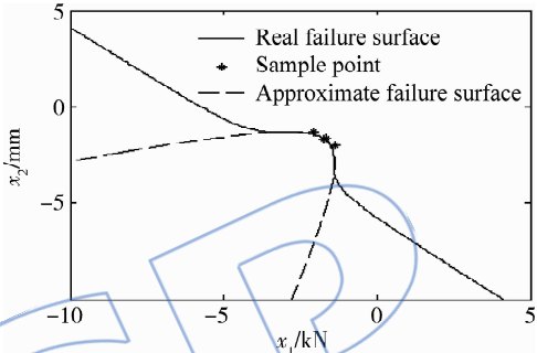
图 7 例 1 择优后结果 Fig. 7 Choosing result of example 1
