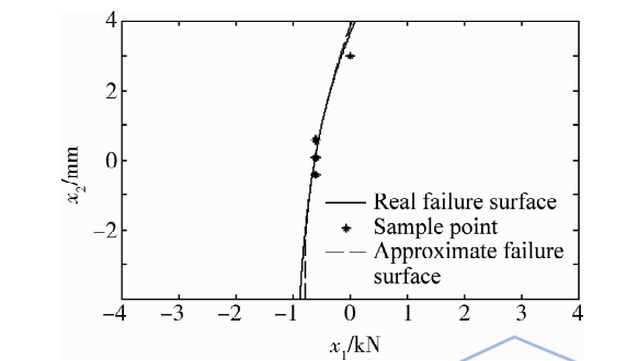
图 9 例 3 择优后结果 Fig. 9 Choosing result of example 3
