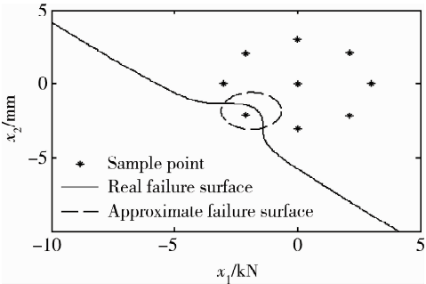
图 3 例 1 第 1 次迭代 Fig. 3 First iterative step of example 1
