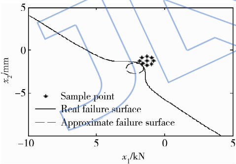
图 4 例 1 第 2 次迭代 Fig. 4 Second iterative step of example 1
