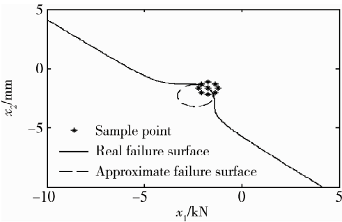
图 5 例 1 第 3 次迭代 Fig. 5 Third iterative step of example 1
