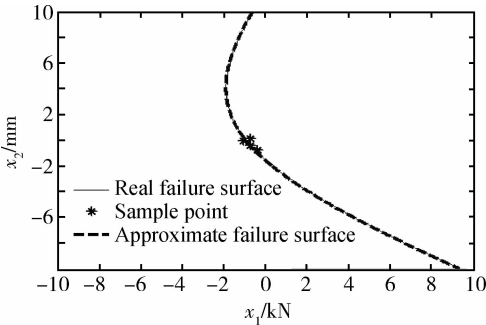
图 8 例 2 择优后结果 Fig. 8 Choosing result of example 2
