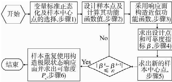
图 2 基于样本重复使用失效响应曲线法 计算流程
